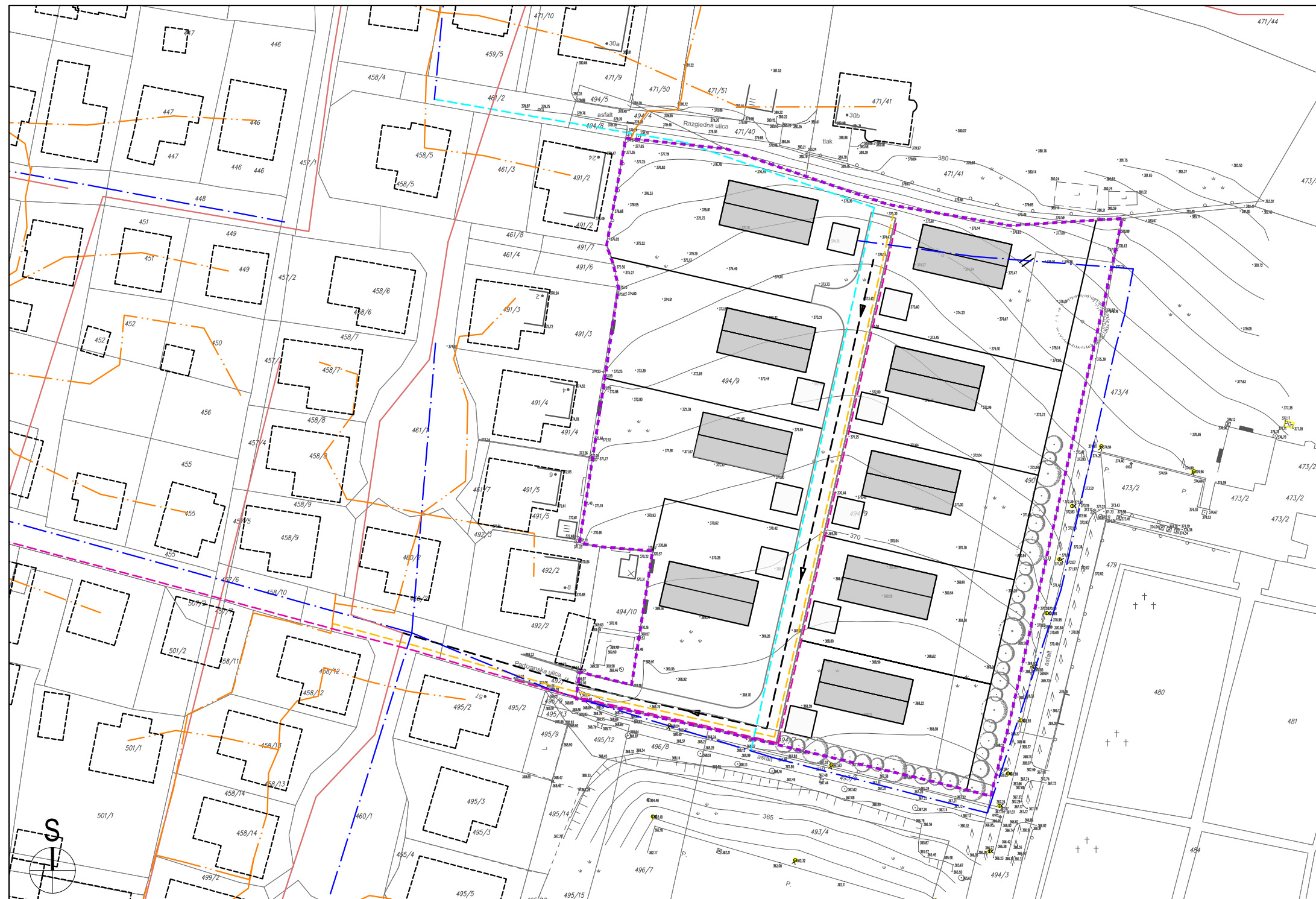
Prikaz priključitve na elektroenergetsko omrežje
