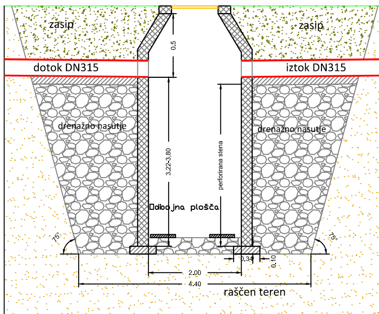
PREREZ A - A:
