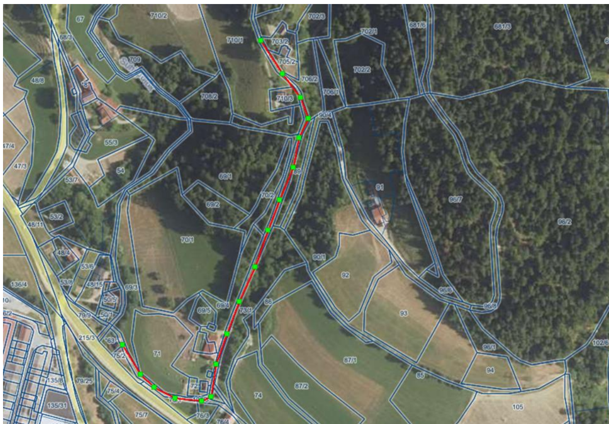
Slika 3: Trasa ceste: JP 846121 G1-Hudej-Podrzavnik-Snežič-Tumpl in JP 846122 Hudej- Podrzavnik v dolžini 550 m
